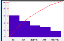
パレート図
