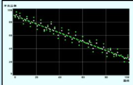
散布図
