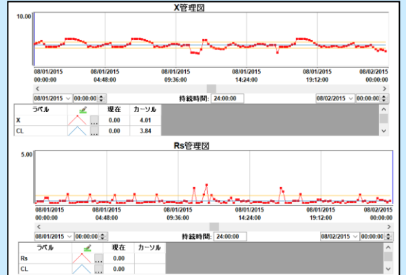
管理図
